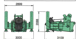
【6】リーダブラケット 10.5ton
